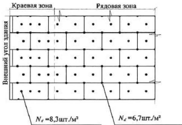
Пример фрагмента теплоизоляции стен выше отм. + 40,0 от уровня отмостки здания
